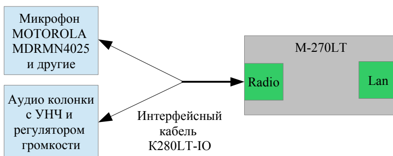
Рис. 9 Схема подключения операторского оборудования к контроллеру М-270LT, при работе интерфейса в режиме «Терминал IO».
