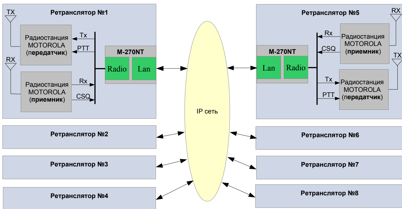
Рис. 16 Схема организации связи при параллельном соединении ретрансляторов.
