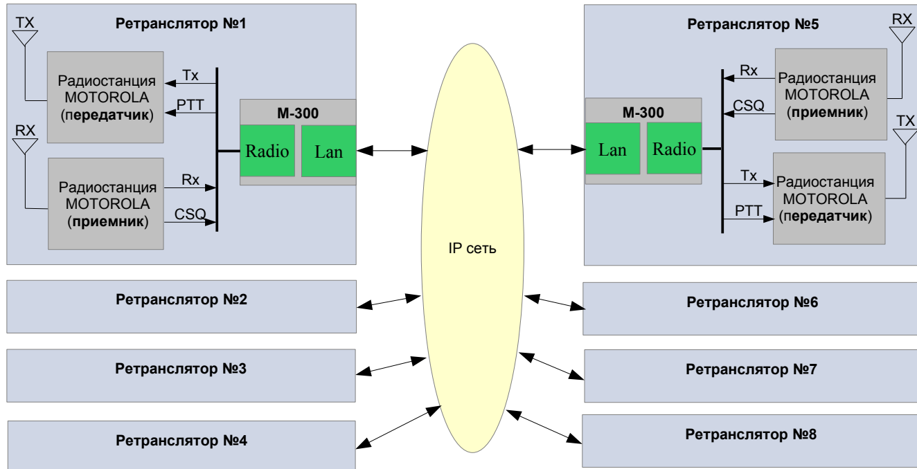
Рис. 3.5.1 Схема организации связи при параллельном соединении ретрансляторов.
